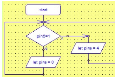
Test conditionnel sur une entrée
